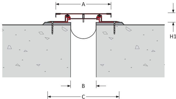
Megatec 600 : A25
